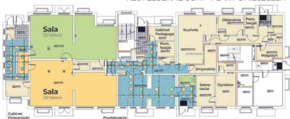
RZUT ŻŁOBKA Z GÓRY - PLAN POMIESZCZEŃ
